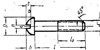
Винт для металла с полукруглой головкой
