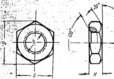
Гайка низкая
