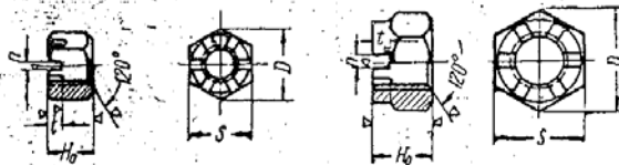
Гайка корончатая
