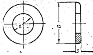
Шайба штампованная
