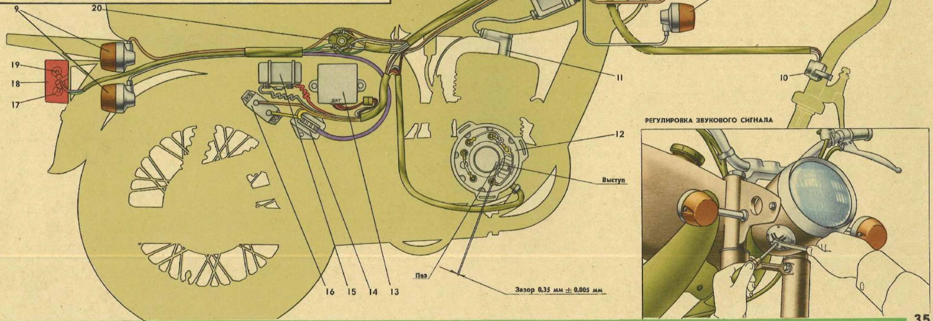
СХЕМА ЭЛЕКТРООБОРУДОВАНИЯ С ЭЛЕКТРОННОЙ СИСТЕМОЙ ЗАЖИГАНИЯ С ГЕНЕРАТОРОМ Г427
