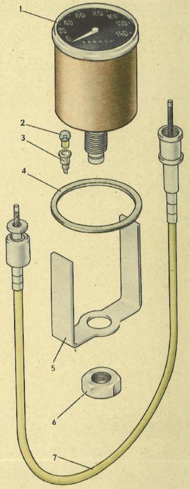
Рис. 32. Спидометр
