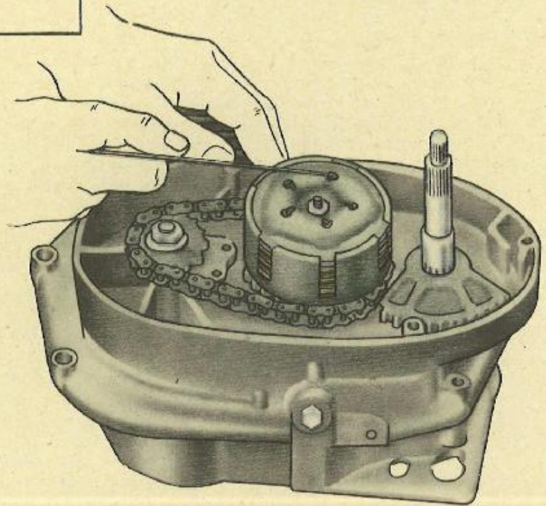
ВЫВОД ПРУЖИН ИЗ НАЖИМНОГО ДИСКА
