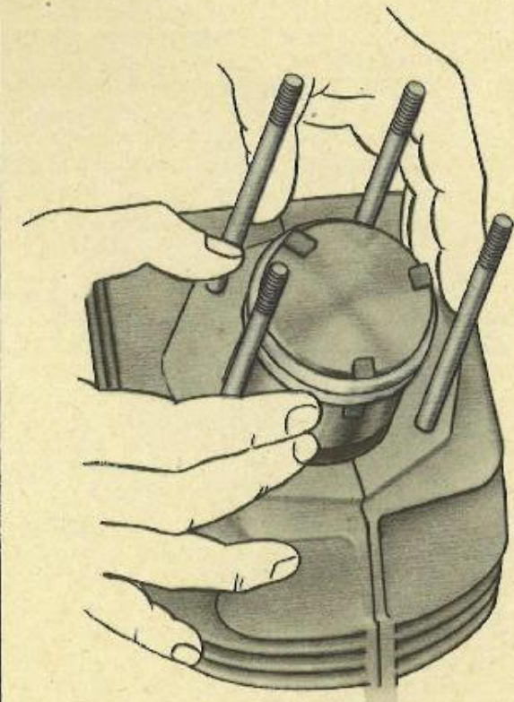
СНЯТИЕ ПОРШНЕВЫХ КОЛЕЦ
