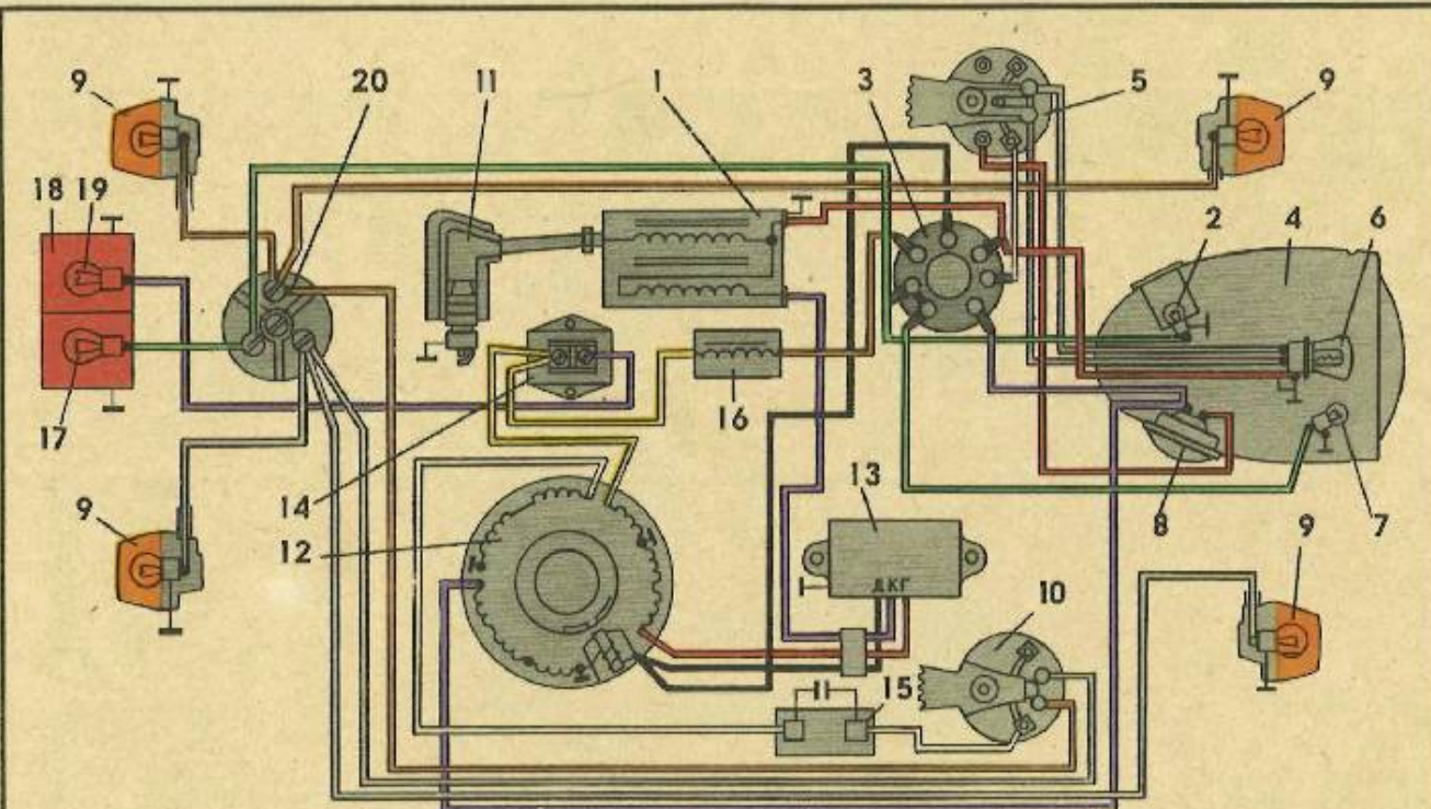
СХЕМА ЭЛЕКТРООБОРУДОВАНИЯ С ЭЛЕКТРОННОЙ СИСТЕМОЙ ЗАЖИГАНИЯ С ГЕНЕРАТОРОМ Г427
