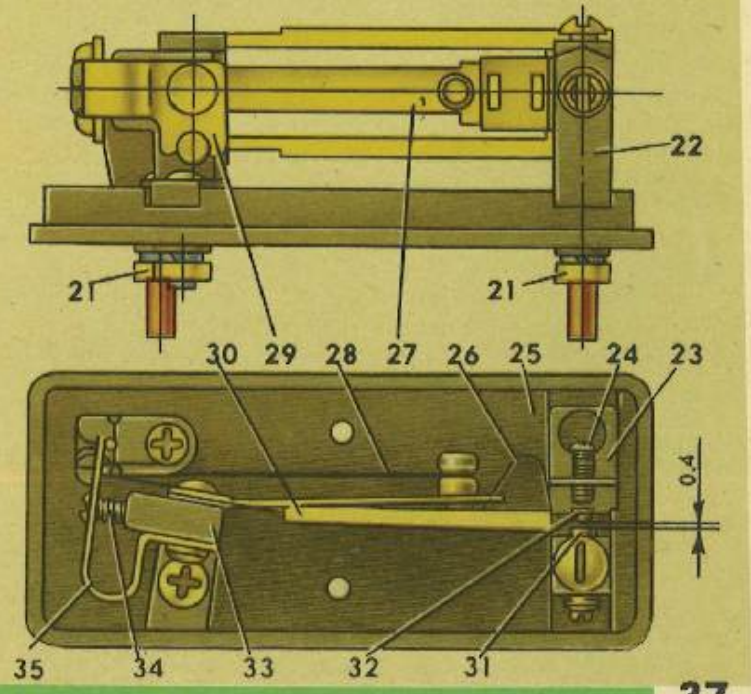
МЕХАНИЗМ ПРЕРЫВАТЕЛЯ УКАЗАТЕЛЕЙ ПОВОРОТА
