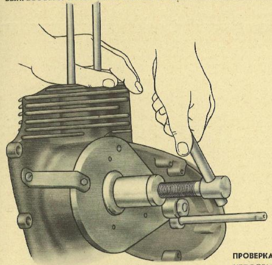
ВЫПРЕССОВКА КОЛЕНЧАТОГО ВАЛА ИЗ ЛЕВОЙ ПОЛОВИНЫ КАРТЕРА
