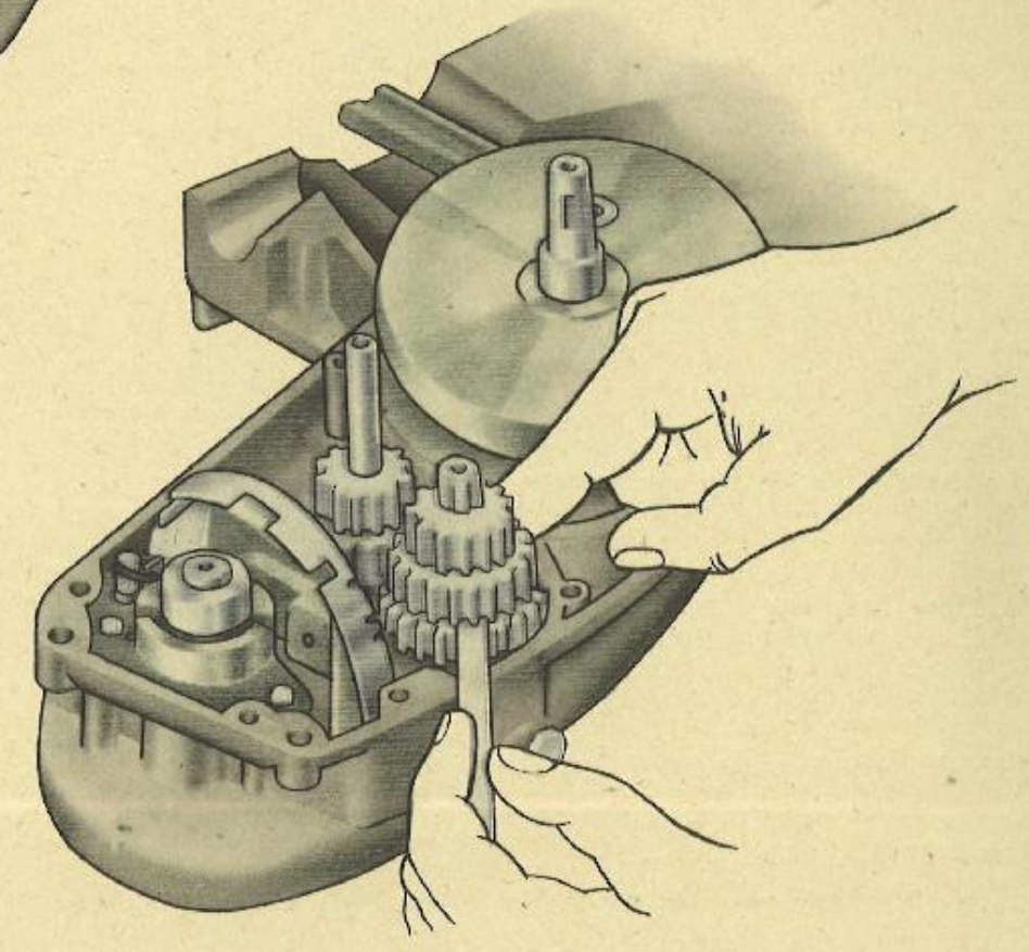
ПРОВЕРКА ЗАЗОРА МЕЖДУ КУЛАЧКАМИ НЕПОДВИЖНОЙ ШЕСТЕРНИ ВТОРОЙ ПЕРЕДАЧИ И ПОДВИЖНОЙ ШЕСТЕРНИ ТРЕТЬЕЙ ПЕРЕДАЧИ
