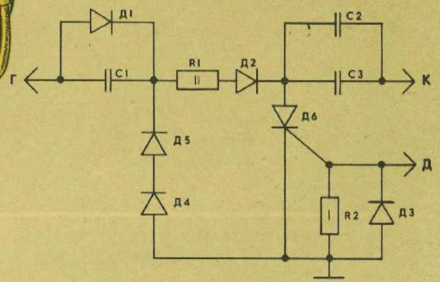
СХЕМА ЭЛЕКТРОННОГО КОММУТАТОРА КЭТ-1А
