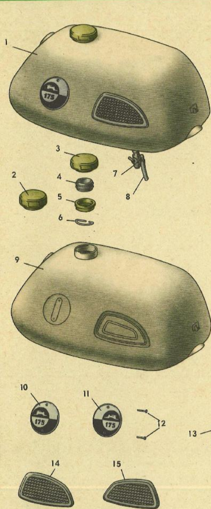
Рис. 4. Бак топливный
