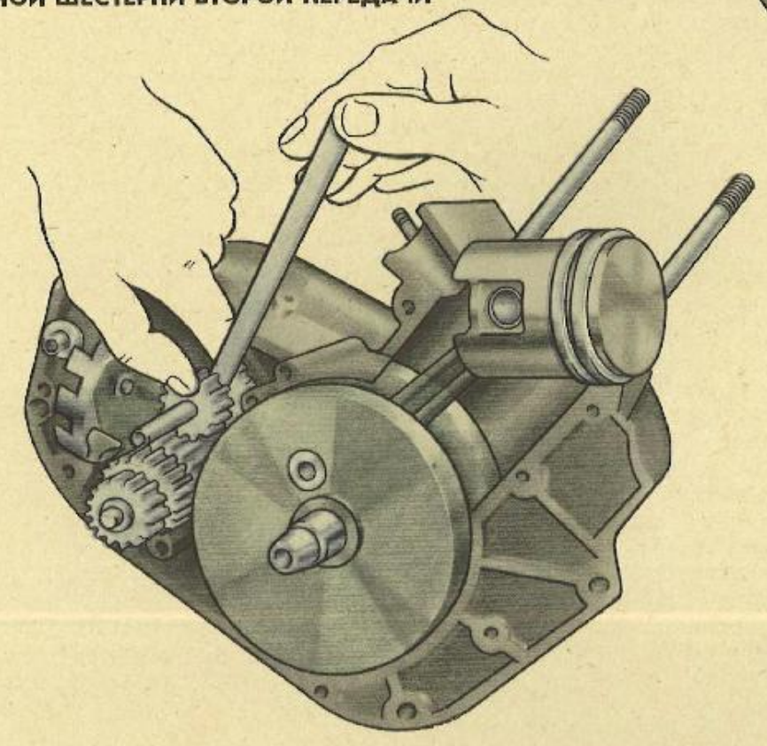
ПРОВЕРКА ЗАЗОРА МЕЖДУ КУЛАЧКАМИ НЕПОДВИЖНОЙ ШЕСТЕРНИ ТРЕТЬЕЙ ПЕРЕДАЧИ И ПОДВИЖНОЙ ШЕСТЕРНИ ВТОРОЙ ПЕРЕДАЧИ
