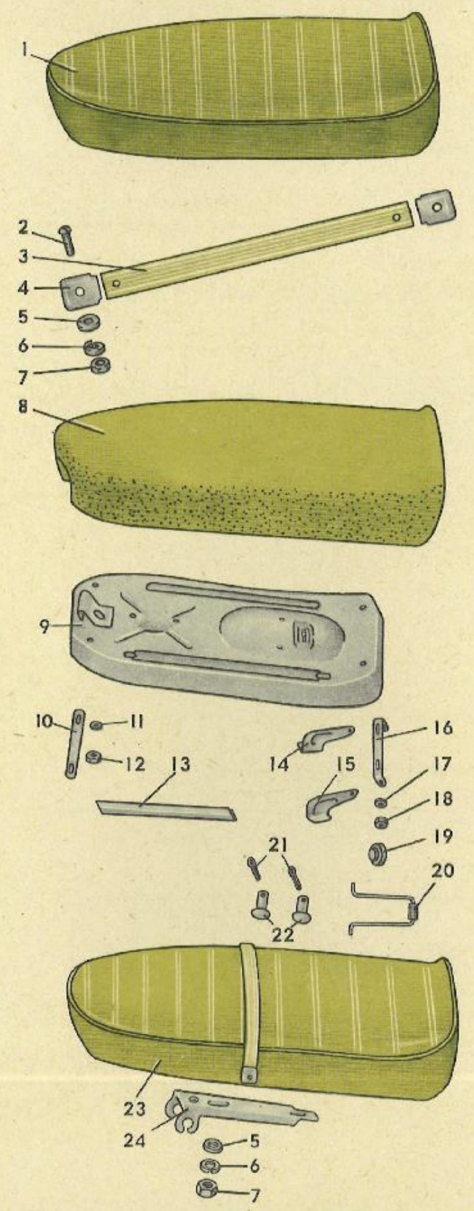
Рис. 19. Седло
