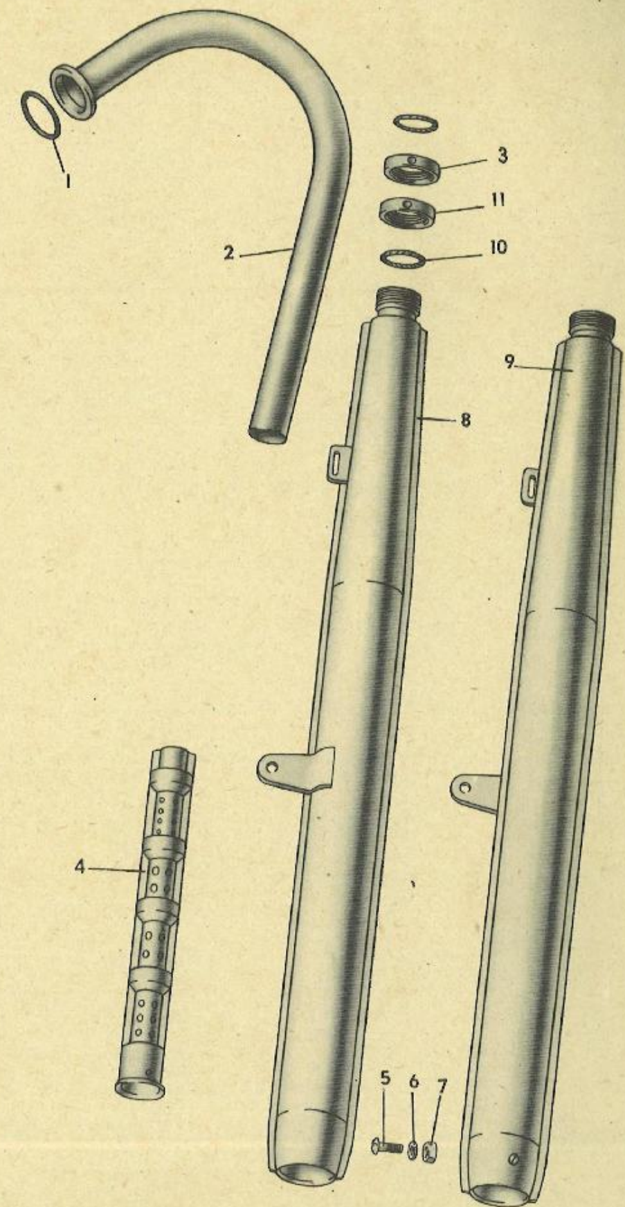
Рис. 6. Система выпуска газа
