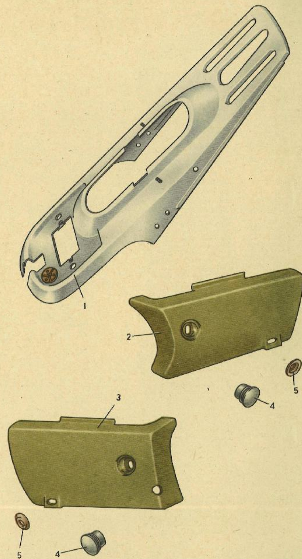
Рис. 27. Закрытия
