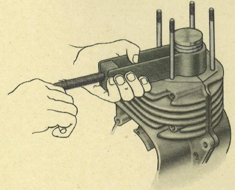
ВЫПРЕССОВКА И ЗАПРЕССОВКА ПОРШНЕВОГО ПАЛЬЦА
