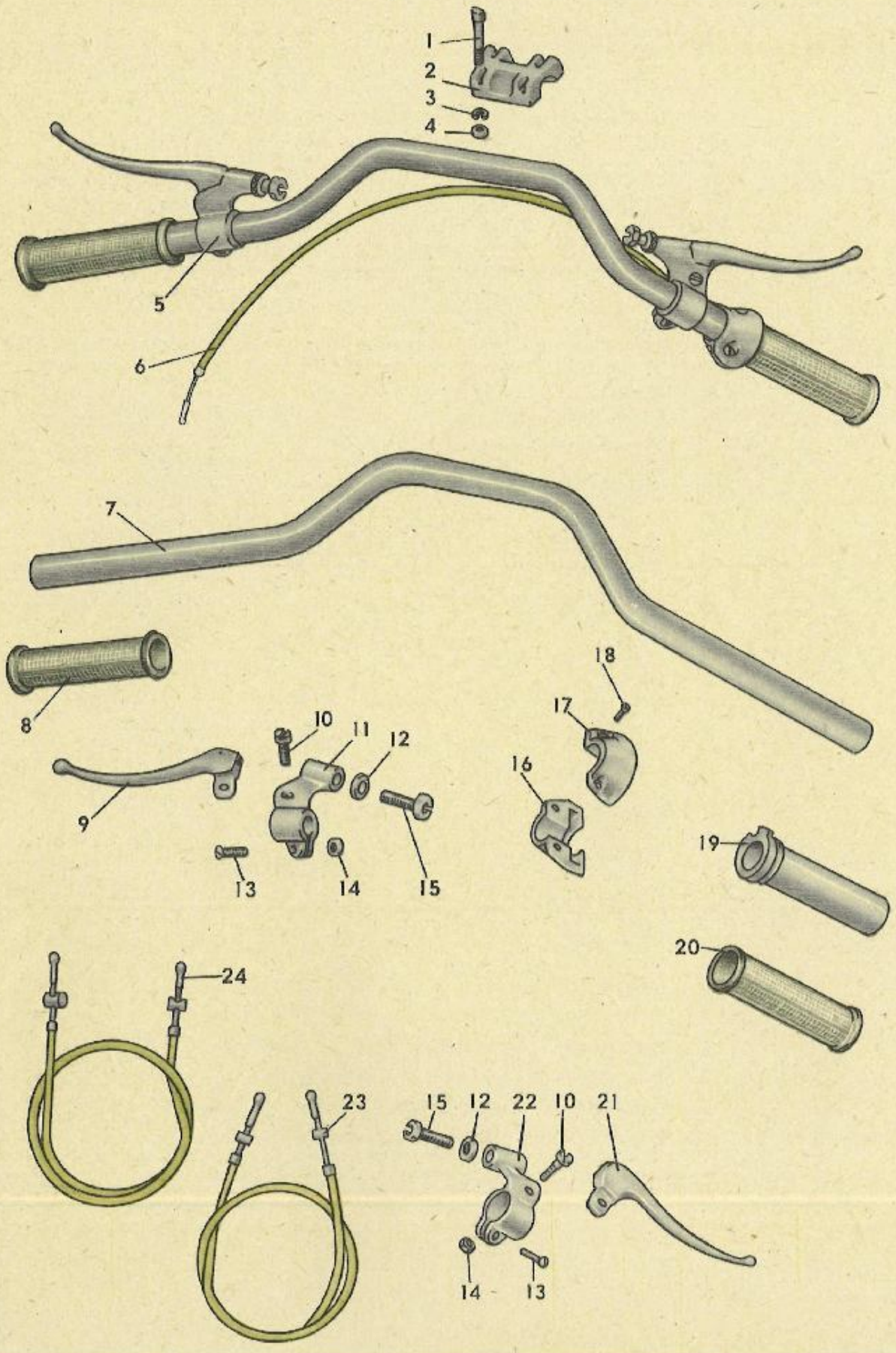
Рис. 18. Руль
